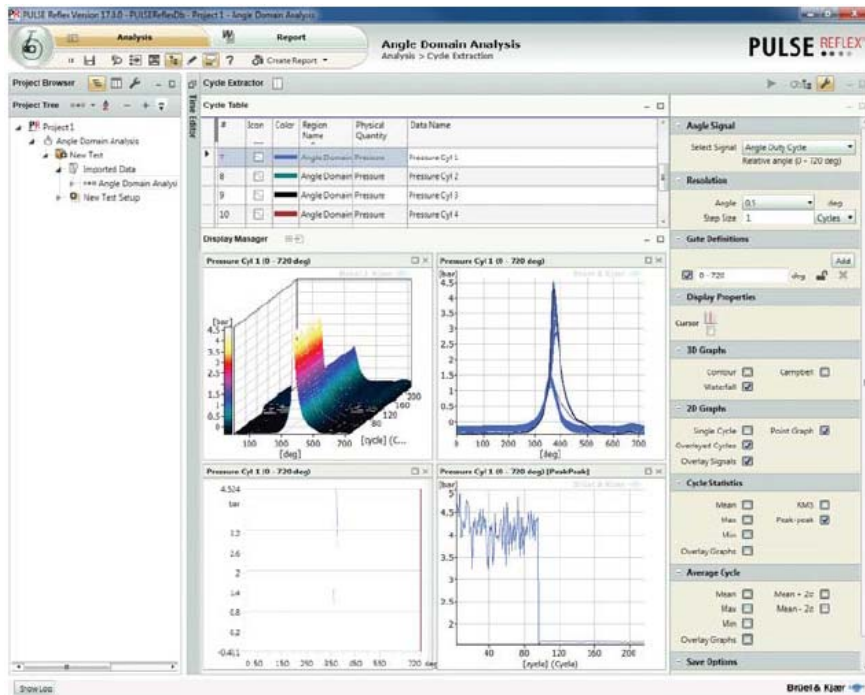
На рис. 3 показано давление в цилиндре, измеренное для бензинового двигателя с отсечкой подачи топлива приблизительно после половины выполненных измерений. Давление в цилиндре было представлено на экране в четырех различных форматах: каскадная диаграмма, 2D-диаграмма с наложением периодов, точечный график* и график размаха†.
