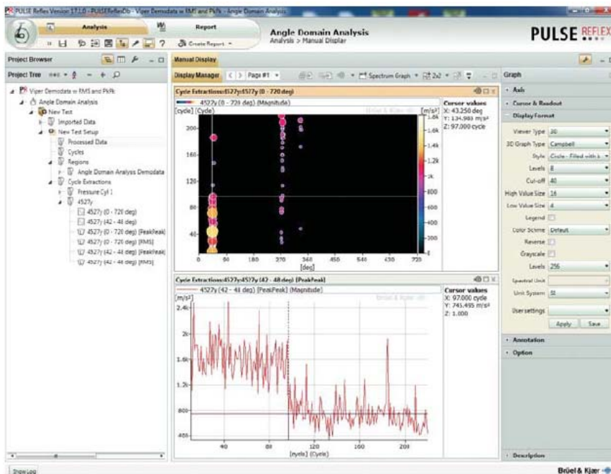
Приложение Reflex Angle Domain Analysis (Анализ в угловом базисе) предлагает для облегчения локализации единичных «событий» в измерении использовать диаграмму Кэмпбелла. Эта диаграмма позволяет обнаружить угловые значения наиболее существенных пиков в сигнале вибрации. На рис. 4. можно видеть, что в области 43° положения коленчатого вала при отсечке топлива исчезают пики, таким образом, изменение вибрации связано с впрыском топлива в цилиндр.
