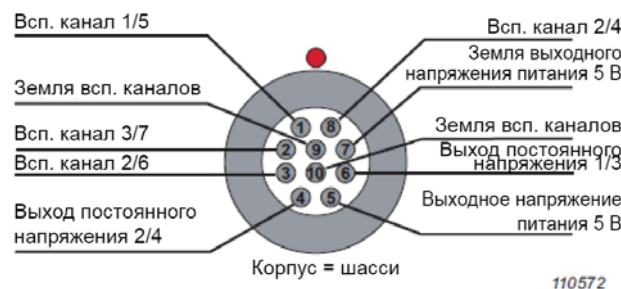
Рисунок 2. 10-контактный соединитель LEMO для подключения вспомогательных каналов
