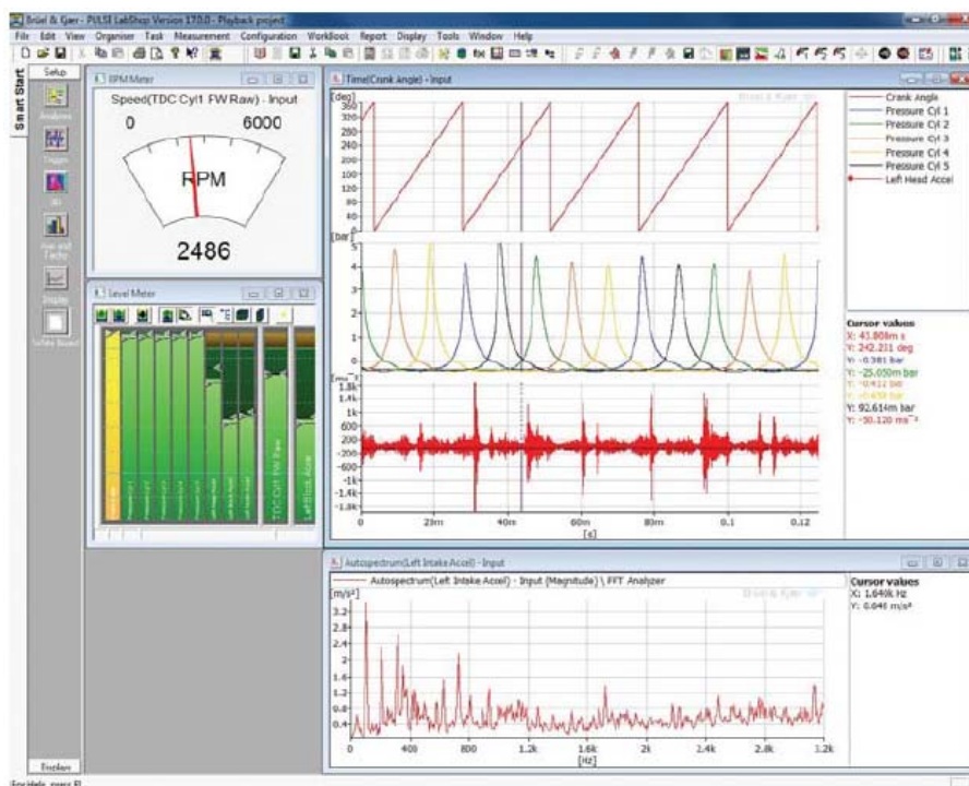
Рисунок 2. Вид типового экрана мониторинга ПО PULSE LabShop в процессе сбора данных. На нем представлен измеритель скорости вращения и уровня по каждому каналу, угловой профиль, сигналы давления в пяти цилиндрах в зависимости от времени и спектральные сигнатуры сигнала вибрации.
