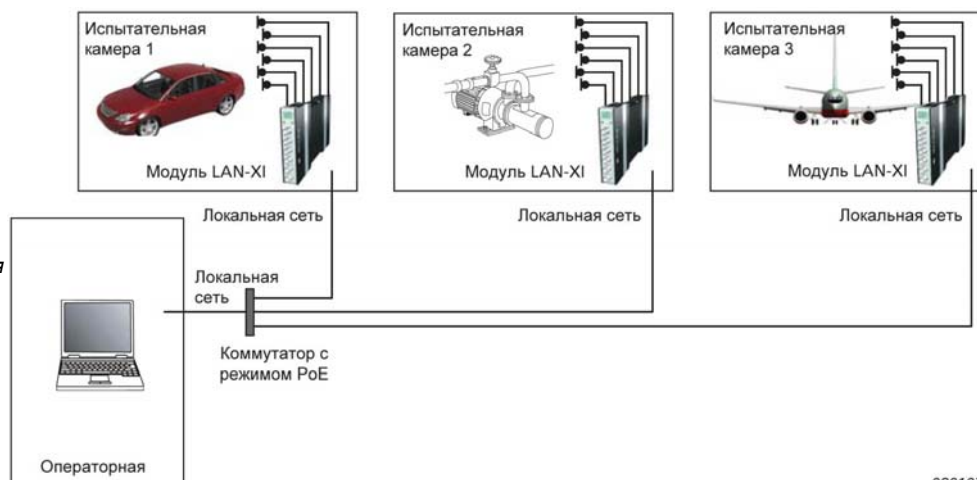
Рис. 1. Применение аппаратуры LAN-XI позволяет значительно уменьшить объем кабельной системы между испытательными стендами и операторной, требуя наличия только сетевых кабелей.
