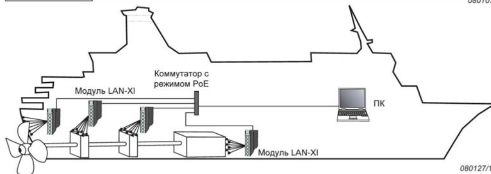
Рис. 2. В распределенной системе, в которой модули расположены непосредственно рядом с объектом испытания, при работе с большими структурами кабельная система датчиков также значительно сокращается.
